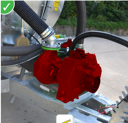
Garda/Julia-pomp: vacuümpomp (pompen) gecombineerd met een centrifugaalpomp (besproeien - 6 bar)
