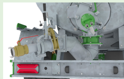
Zuig-/afvoerafsluiter , snelkoppeling voor Ø 150 mm slangen of brandweeraansluiting.
