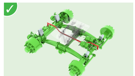
Bogie met lastafhankelijk remsysteem
