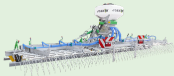
Scariflex R6S5 (6 uitvoeringen) Ideale beluchter voor weiden met één rij nivelleerbladen.
