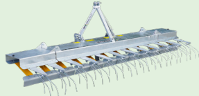
BF (10 uitvoeringen) Eenvoudige machine om gemakkelijk te beluchten en koeienmest te verspreiden.
