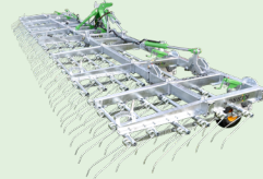
Scariflex R6S6 (7 uitvoeringen) Beluchter voor grasland en halfharde grond.
