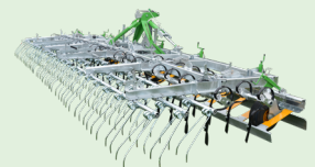
Scariflex R6D2S3 (2 uitvoeringen) All-in-one beluchter (molshopen afvlakken en beluchten).
