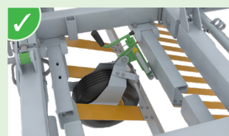
Positionnement des roues idéal pour un bon suivi du terrain.
