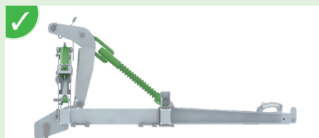
Châssis porteur tubulaire indépendant couplé à un attelage articulé et un 3 e point sur ressort afin d'avoir un suivi du terrain souple.
