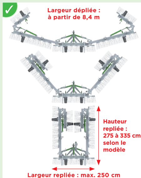
Repliage hydraulique double pour les modèles à partir de 8,4 m de largeur de travail.
