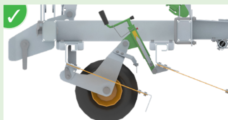
Réglage de la hauteur des roues à l'aide d'une manivelle. Graduation et flèche de repérage.
