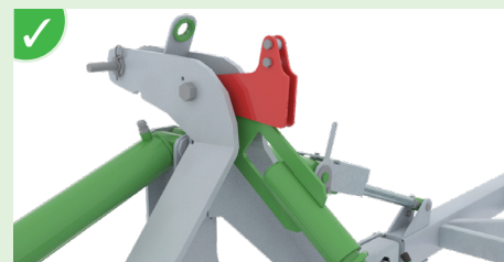
Blocage du 3 e point sur ressort pour une bonne stabilité sur route (modèles : 7,2 à 12 m).
