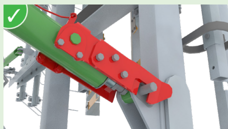
Blocage hydraulique et mécanique des allonges pour une sécurité maximale sur la route.
