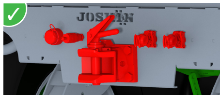
Komplet gniazd do oświetlenia, hamulców i wywrotu drugiej przyczepy z zaczepem tylnym obrotowym.
