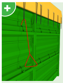
Hak do łatwego mocowania plandeki, nawet w przypadku wyższych skrzyni.
