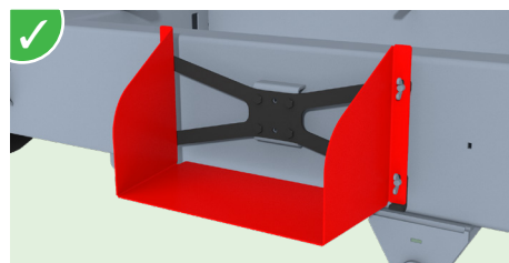
Rylna zsympowa do spustu zbożowego (440 x 240 mm) mocowana pod skrzynią.
