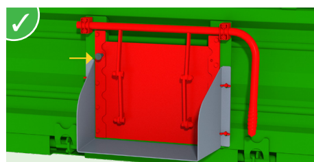
Duży spust zbożowy (otwór: 390x300 mm) z automatyczną blokadą.
