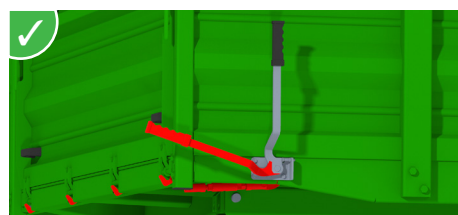
Regulowany system blokowania z przekładnią systemu ryglowania haków burt bocznych i tylnych w celu zapewnienia prawidłowego docisku do uszczelki.
