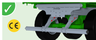
Regulacja wysokości tylnego zderzaka z ustawianiem kilku pozycji
