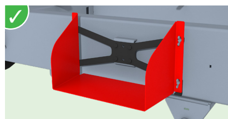
Pico vertedor para escotilla para granos (440x240 mm) con almacenamiento debajo de la caja.
