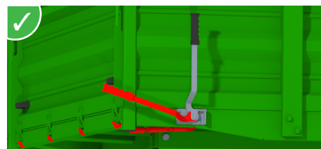
Sistema de bloqueo ajustable con gran palanca de ganchos en los adrales laterales y trasero para garantizar un correcto apoyo en las juntas.
