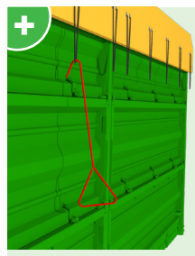
Haken zum einfachen Befestigen der Plane, auch bei höheren Seitenwänden.
