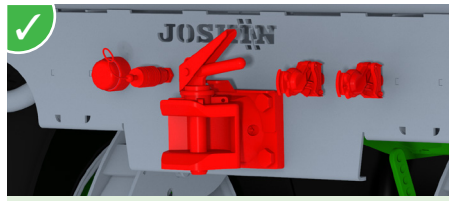
Vollständige Anschlüsse für die Beleuchtung, das Bremssystem und zum Abkippen eines zweiten Anhängers mit hinterem drehbarem Zugmaul.
