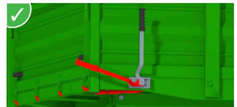
Einstellbares Verriegelungssystem mit einer sehr hohen Übersetzung der Haken an den Seiten- und Heckwänden, um eine korrekte Auflage auf die Dichtungen zu gewährleisten.
