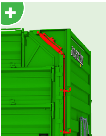
Doppelte hydraulische Verriegelung der Heckklappe mit Dichtung und eingebauter mechanischer Verriegelung.
