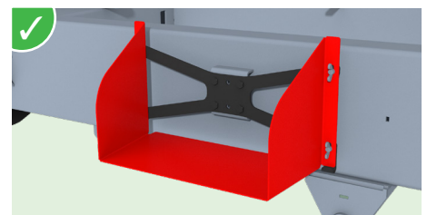
Entladerutsche für Getreideluke (440x240 mm) mit Ablage unter dem Kasten.
