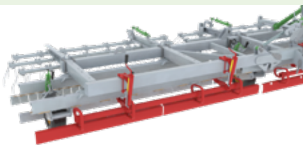
Unabhängige Planierschienen , die je nach Modell unterschiedlich breit sind (90 bis 130 cm) und vor den Rädern angebracht sind, um das Gelände zu ebnen.
