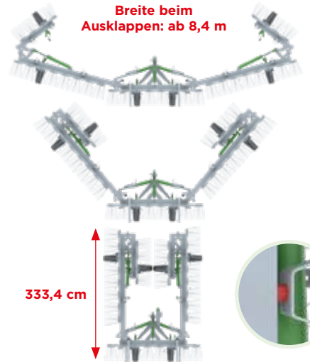
Doppeltes, hydraulisches Einklappen mit verstellbarem Anschlag und geräuschkämpfendem Ertalon für Modelle ab 8,4 m Arbeitsbreite.
