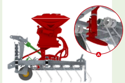
Druckluftsämaschine (150, 300 oder 450 l) mit elektrischem Antrieb. Verschiedene Streuer möglich (max. Ø der Körner: von 2,5 bis 7 mm). Vorausrüstung möglich bei den Modellen 480, 600, 720 und 960. (A) Prallbleche (8 oder 12, je nach Modell).
