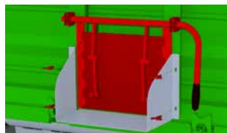
Gran escotilla para granos (apertura: 390x300 mm) con pico vertedor.
