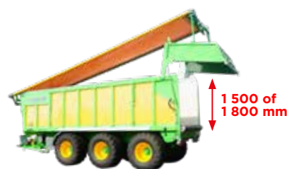
TELECOVER dekzeil (hermetisch) , met een enkel vast opzetschot van 250 mm aan de rechterzijde.
