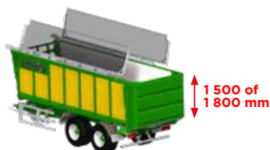
DUO-COVER (2 afdekkingen met net, speciaal voor kuilvoer) , alleen met opzetschotten A B C D .
