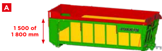
Mechanische opzetschotten met 4 posities (50 - 250 - 400 - 550 mm), met individuele verstelling voor alle 4 zijden.
