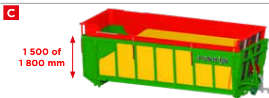
4 hydraulische opzetschotten met meerdere posities van 50 tot 550 mm (afzonderlijk inschuifbaar).
