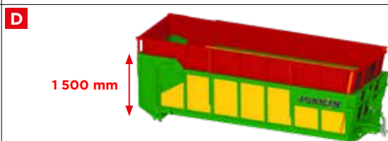
4 hydraulische opzetschotten met meerdere posities van 50 tot 850 mm (afzonderlijk inschuifbaar).
