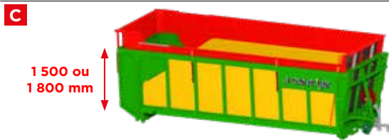
C 4 rehausses hydrauliques multi-positions de 50 à 550 mm (rétractables individuellement).
