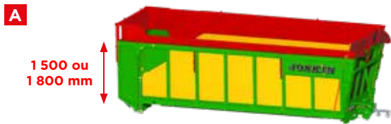
A Rehausses mécaniques 4 positions (50 - 250 - 400 - 550 mm), avec réglage individuel pour les 4 côtés.
