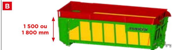
B Rehausses hydrauliques latérales de 50 à 550 mm rétractables individuellement - vantail avant rabattable manuellement - partie arrière mécanique 4 positions.
