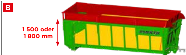
Hydraulische Seitenaufsätze von 50 bis 550 mm einzeln einziehbar - Frontaufsatz manuell abklappbar - mechanischer Hinterteil 4 Positionen.
