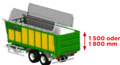
DUO-COVER (2 flexible Netzabdeckklappen, speziell für Silage) , nur mit Aufsätzen A B C D lieferbar.
