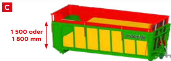
4 hydraulische Mehrpositionsaufsätze von 50 bis 550 mm (einzeln einziehbar).
