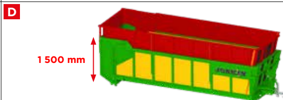
4 hydraulische Mehrpositionsaufsätze von 50 bis 850 mm (einzeln einziehbar).
