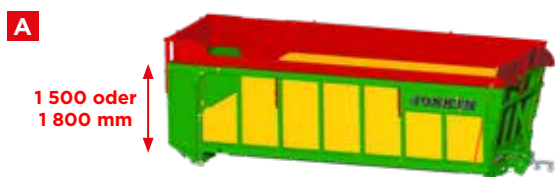
Mechanische Aufsätze mit 4 Positionen (50 - 250 - 400 - 550 mm), mit individueller Einstellung für alle 4 Seiten.
