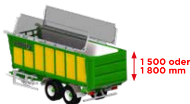
DUO-COVER (2 flexible Netzaabdeckklappen, speziell für Silage) , nur mit Aufsätzen A B C D lieferbar.
