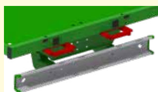
WAGO galvanizados y pintados 2 opciones de tensores de correa en la parte trasera de las plataformas
