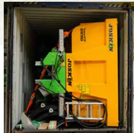
2 przyczepy KTP 22/50 w jednym kontenerze 40 ft HC
