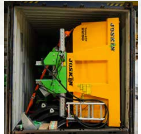
2 przyczepy KTP 22/50 w jednym kontenerze 40 ft HC
