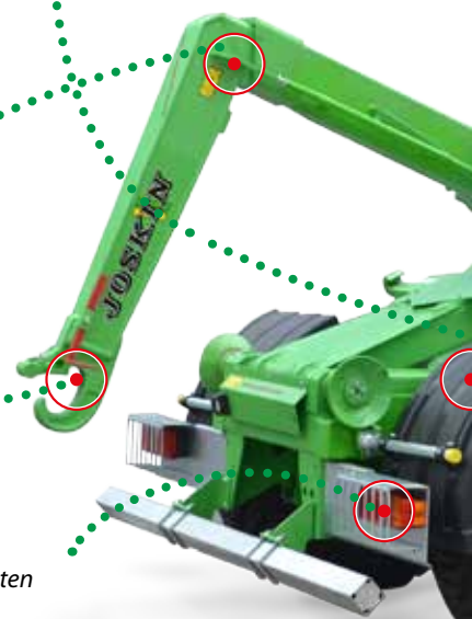
thermoplastische Kotflügel
